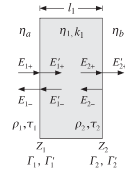
Fig. 5.4.1 Single dielectric slab.
